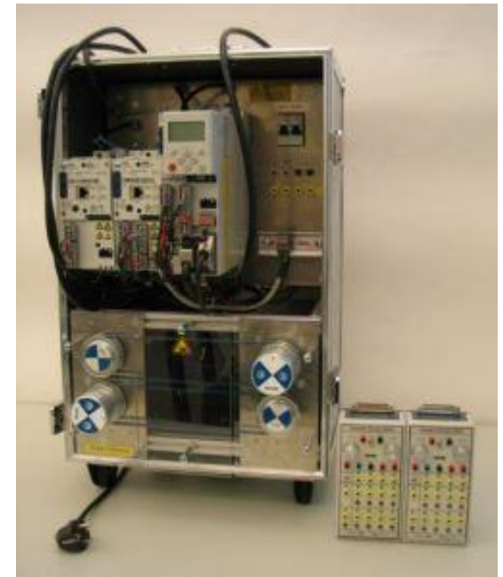
La valise 8400 contient 3 variateurs 8400 StateLine, HighLine et TopLine pour correspondre au mieux au matériel installé sur la machine.
